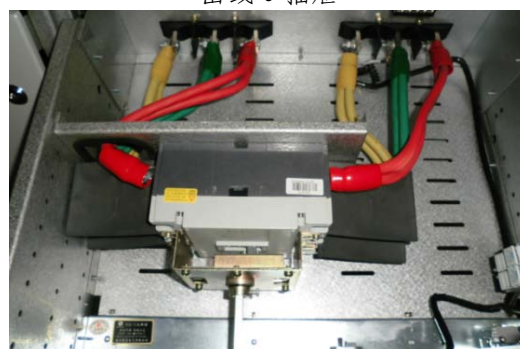
出线 5 抽屉照片
