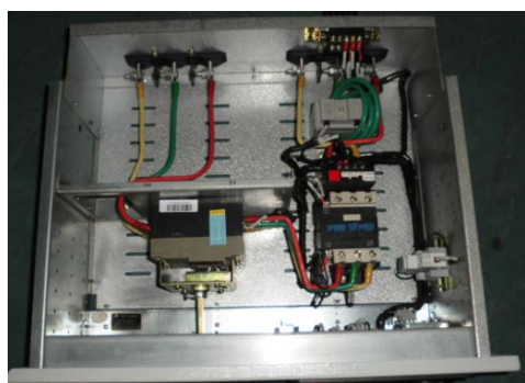
出线 4 抽屉照片
