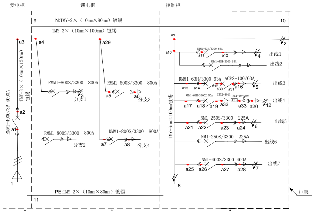
温升、短路点示意图 F1:
